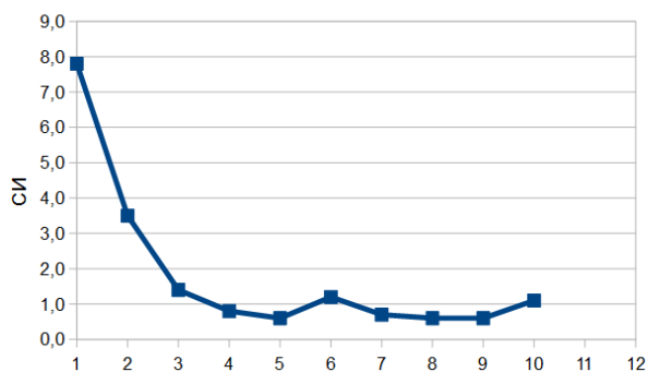
Рис. 14 — Годовой ход СИ и НП
