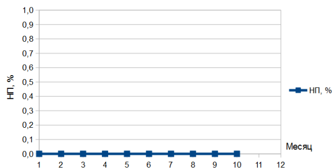
Рис. 16 — Годовой ход СИ и НП
