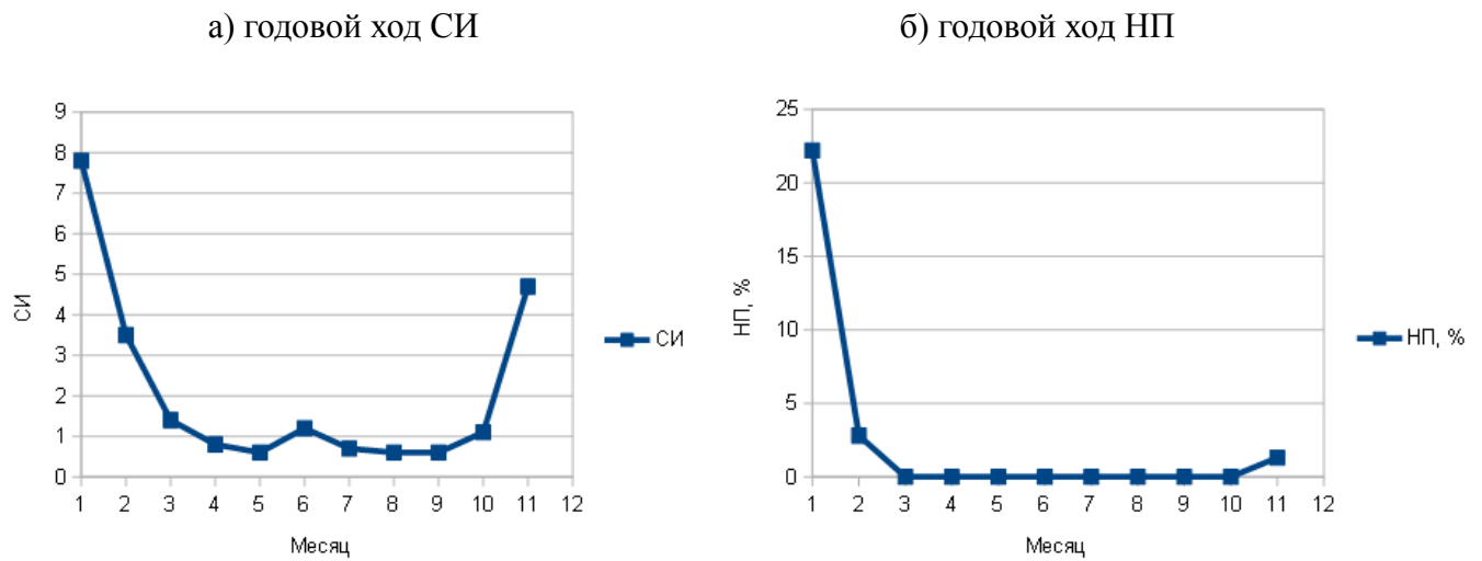
Рис. 14 — Годовой ход СИ и НП
