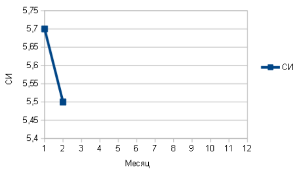
Рис. 4 — Годовой ход СИ и НП
