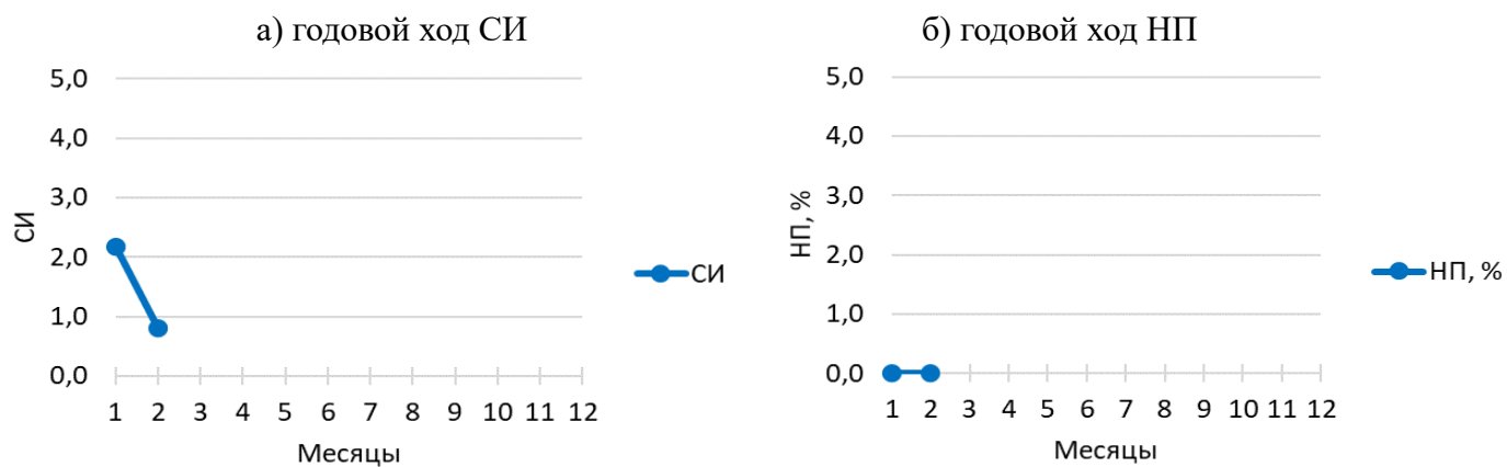
Рис. 16 — Годовой ход СИ и НП
